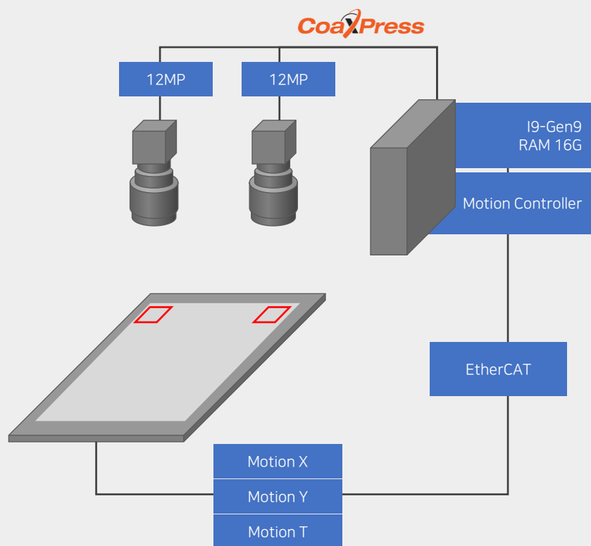
시스템 구성도
